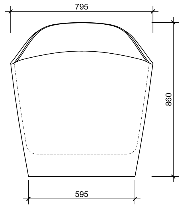
Mặt Đứng
