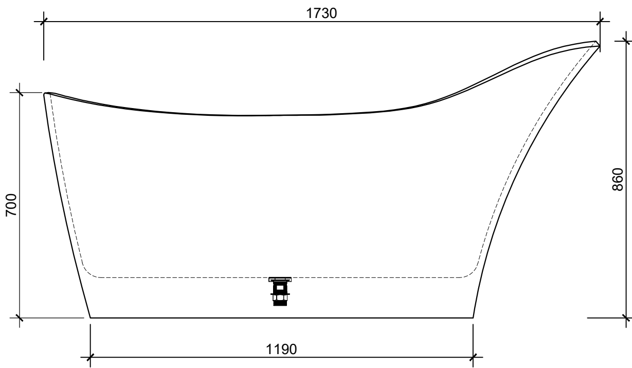
Mặt Đứng
