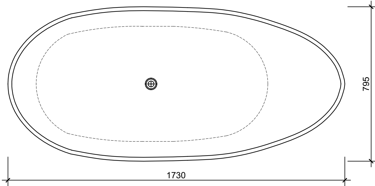
Mặt Bằng
