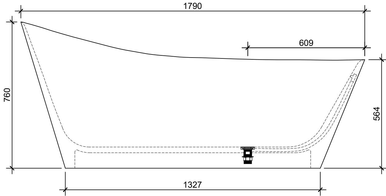
Mặt Đứng
