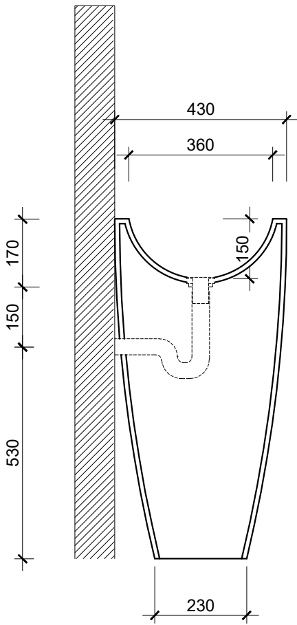
MẶT CẮT
