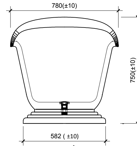
MẶT BÊN
