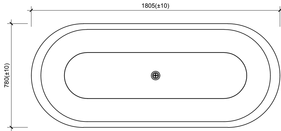
MẶT BẰNG
