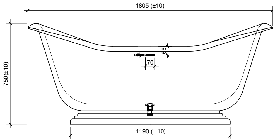
MẶT ĐỨNG
