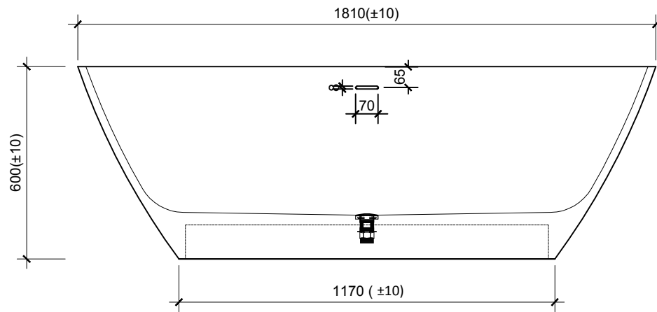
MẶT ĐỨNG
