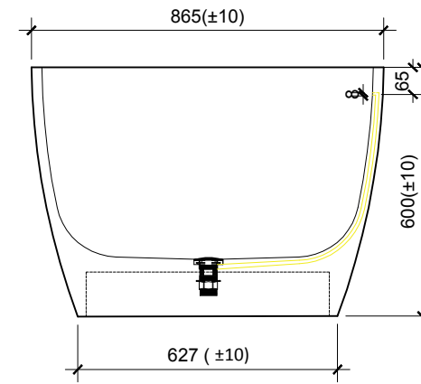
MẶT BÊN
