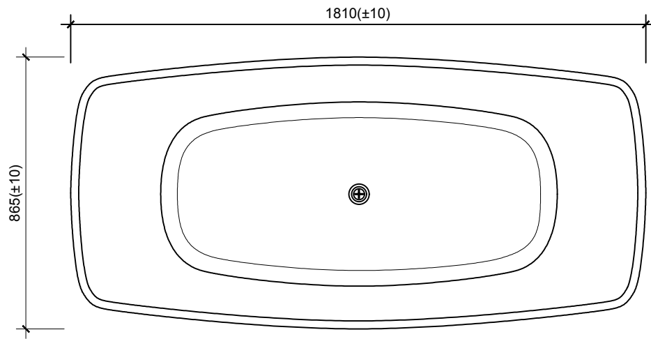
MẶT BẰNG
