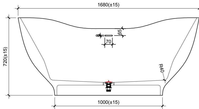
MẶT ĐỨNG
