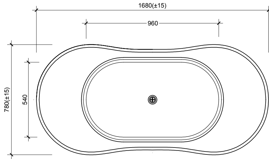
MẶT BẰNG
