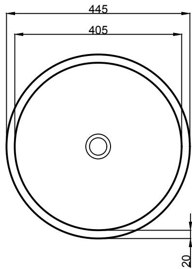
MẶT BẰNG
