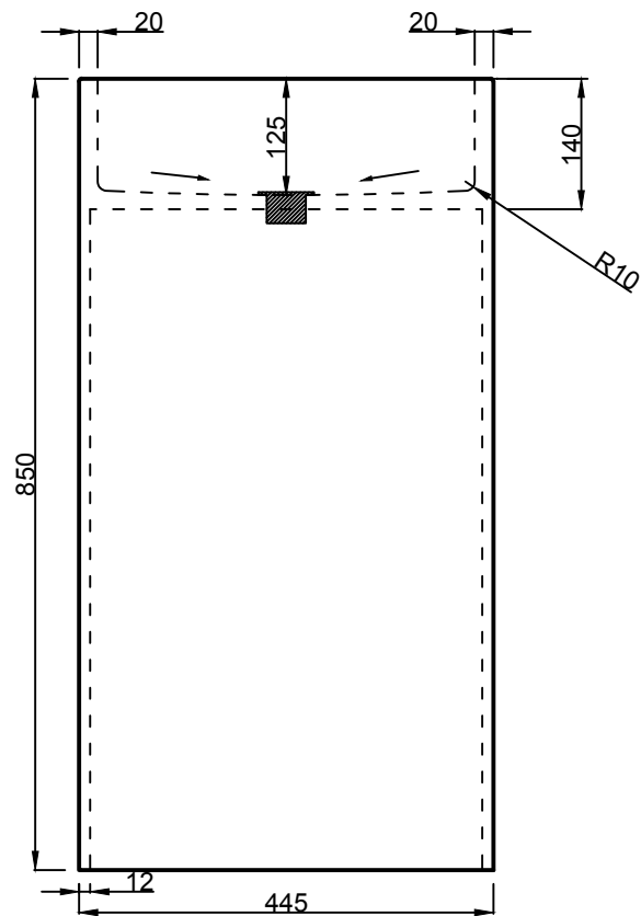
MẶT ĐỨNG
