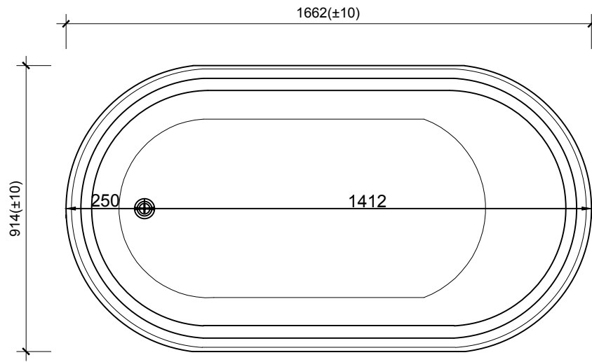
MẶT BẰNG
