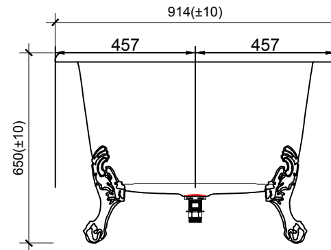
MẶT BÊN
