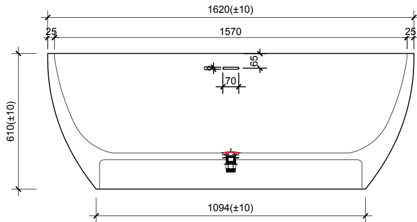
MẶT ĐỨNG
