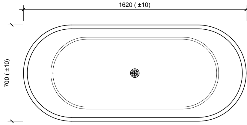
MẶT BẰNG
