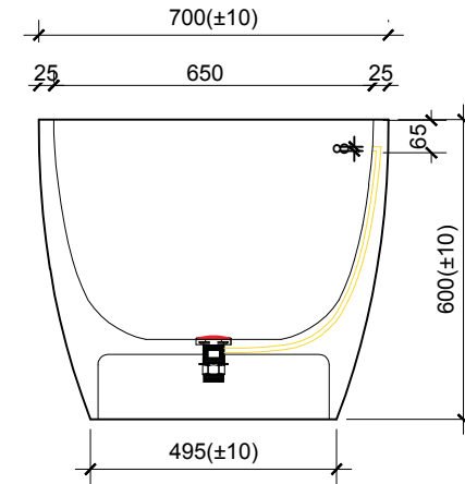
MẶT BÊN
