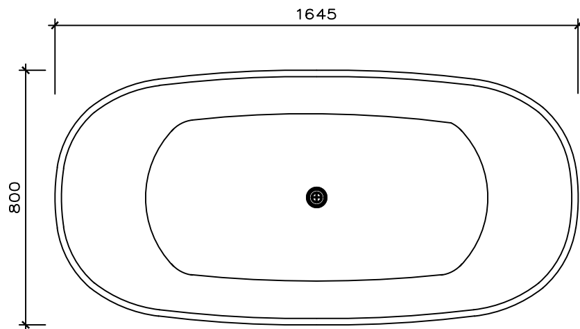
MẶT BẰNG
