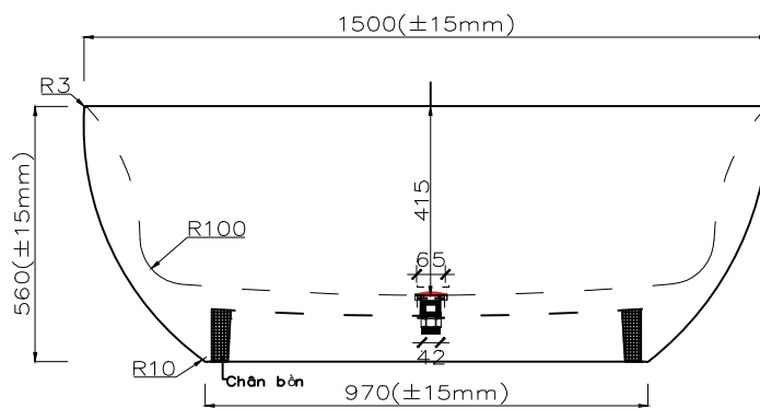
MẶT ĐỨNG
