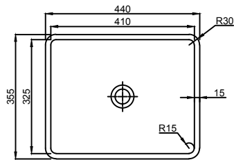
MẶT BẰNG
