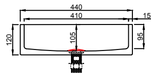
MẶT ĐỨNG
